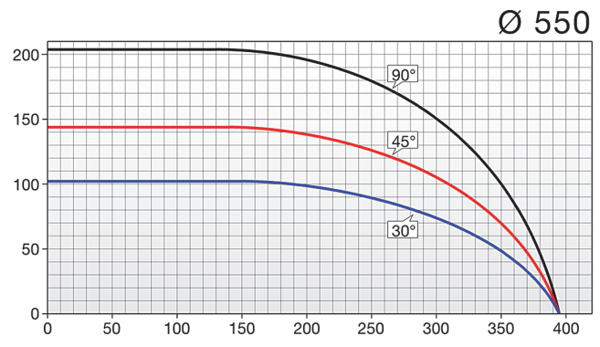
切割曲线图
