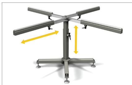
Støtteflade med mulighed for udtræk og forøgelse af højden 03
