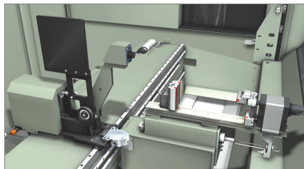
Posizionatore morse 01
