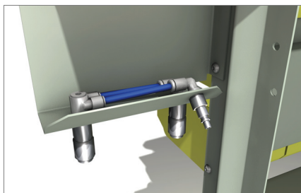
Instalacja sprężonego powietrza 03
