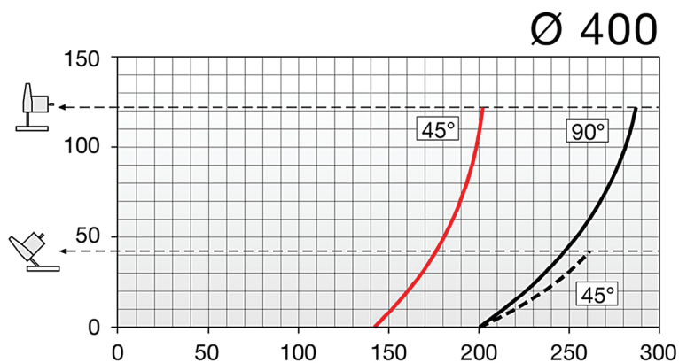
Diagramma di taglio
