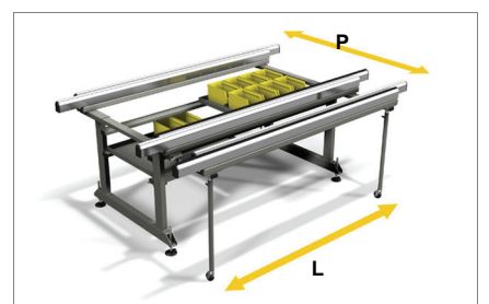
Plano de apoio extensível e alongável 05
