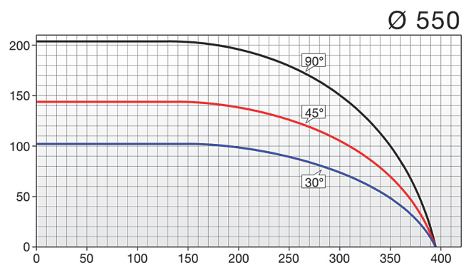
Диаграмма резки
