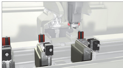
Mordazas motorizadas 01
