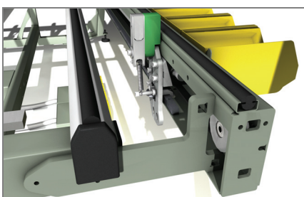
Självcentrerande låsning av karmen 03
