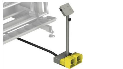
Kontroll och fotpedalssats 02
