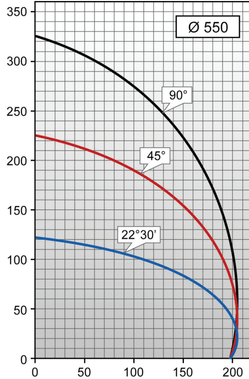
Kesim diagramı
